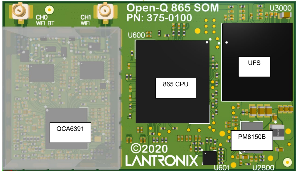
Figure 2 – Open-Q 865XR SOM Top View
