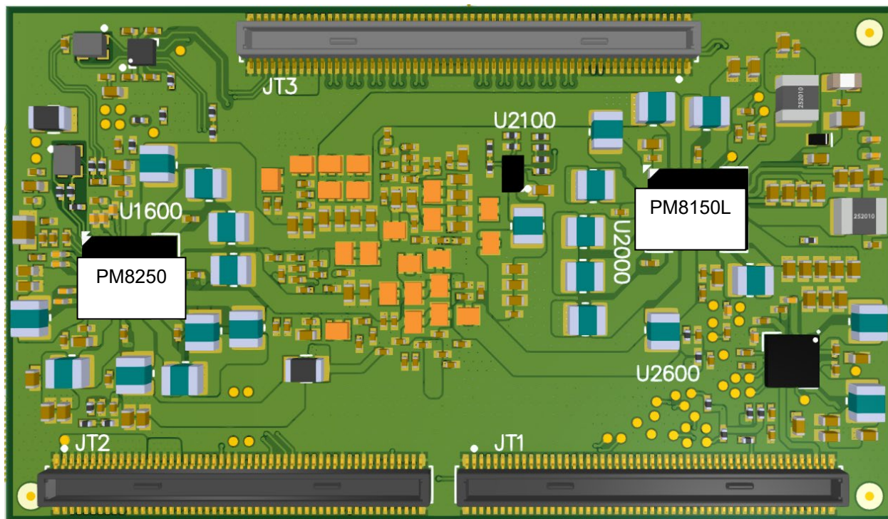
Figure 3 – Open-Q 865XR SOM Bottom View
