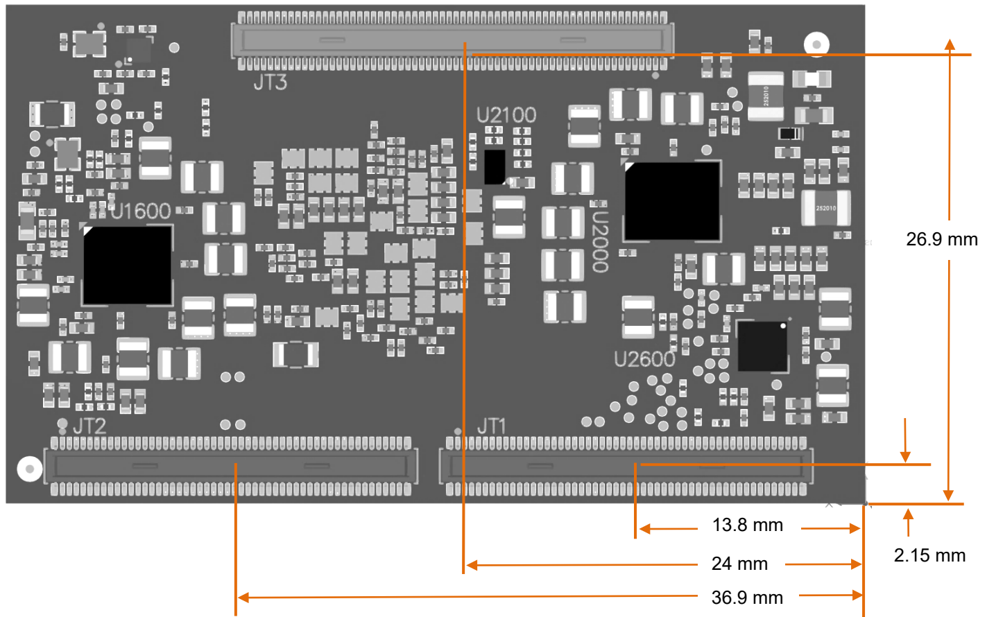
Figure 7 - SOM Land-Pattern Dimensions (mm)
