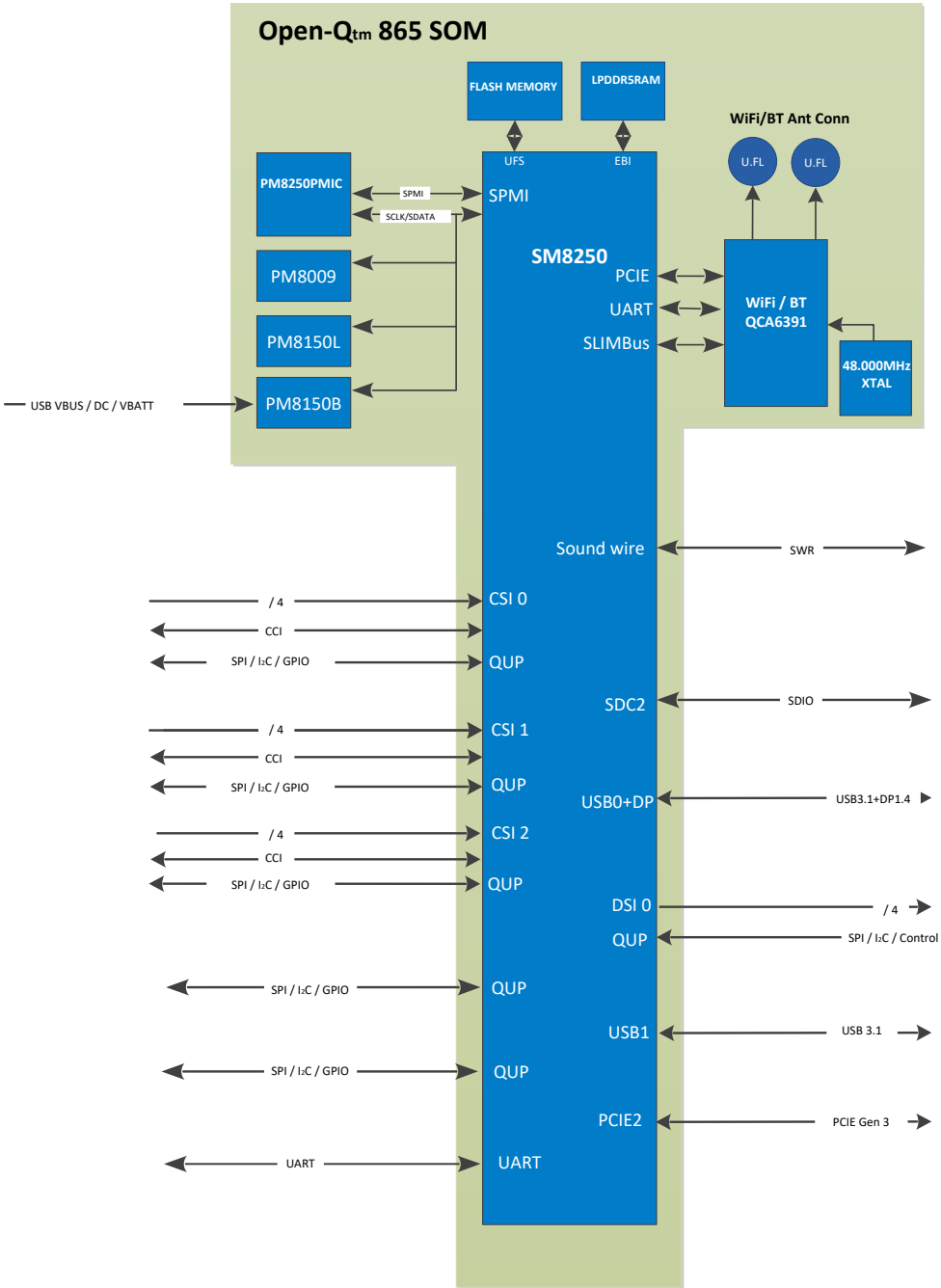
Figure 1 – Open-Q 865XR SOM Block Diagram
