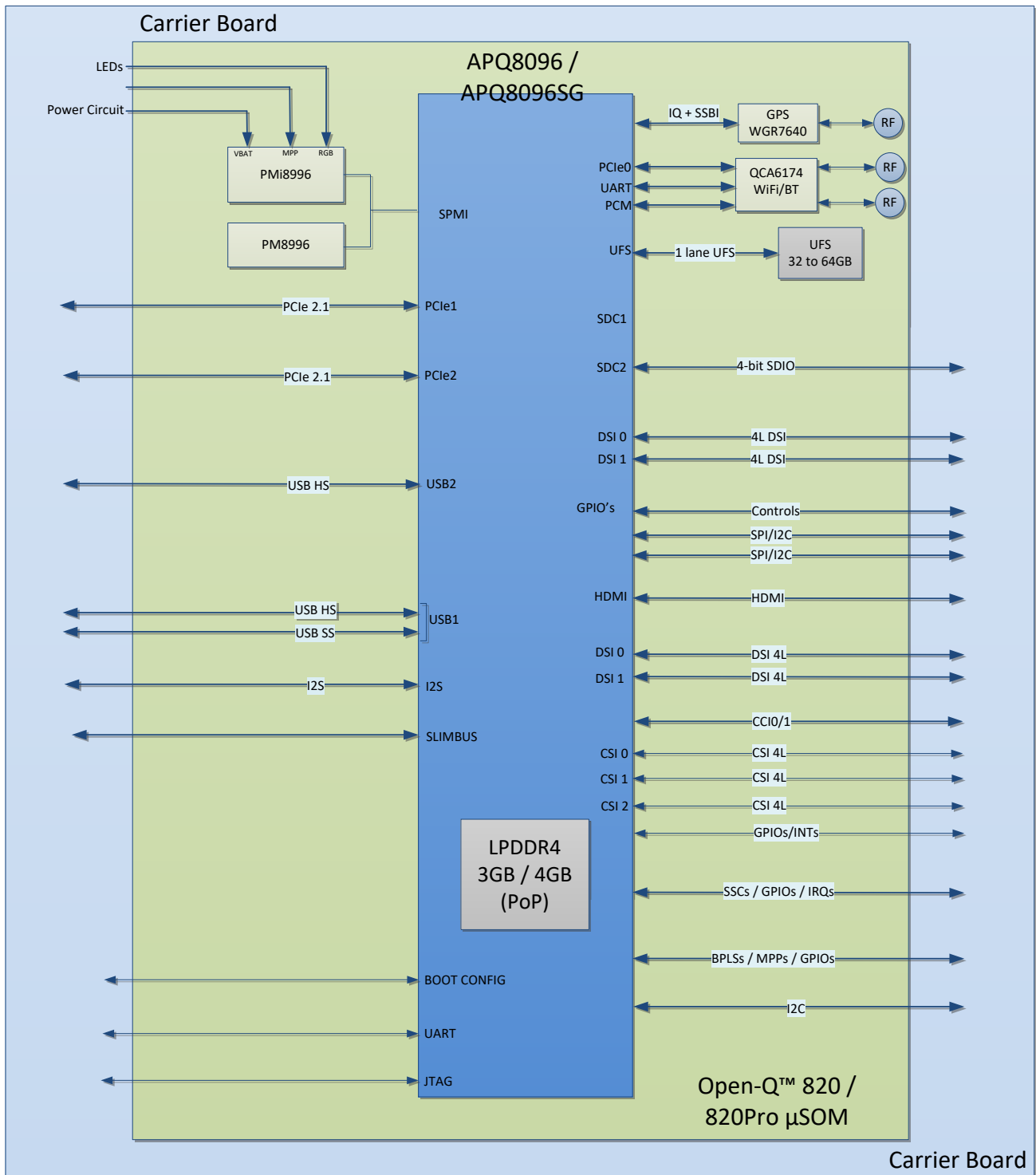
Figure 4 \mu SOM Block Diagram
