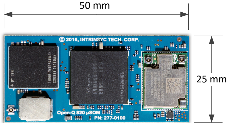
Figure 3 Open-Q 820 / 820Pro \mu SOM
