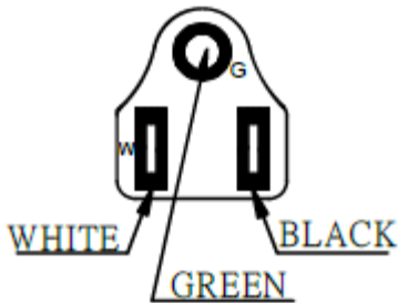
NEMA 5-15P
